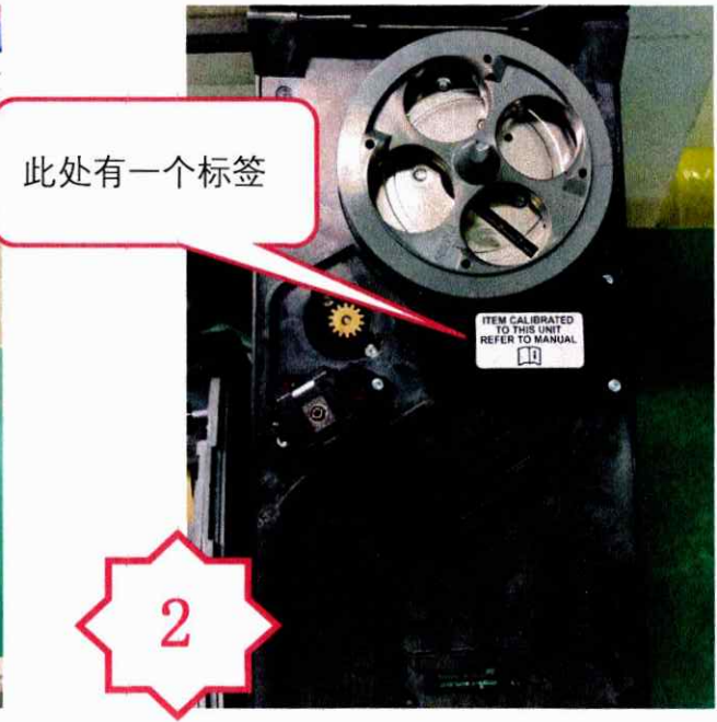
图二，在 Twin Coin Feeder PM1137 塑胶件上有一个 LB2080 或 LB2152 标签
